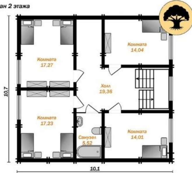
План 2 этажа
