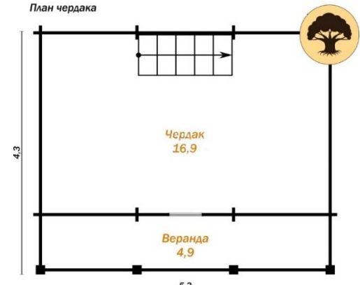
План чердака
